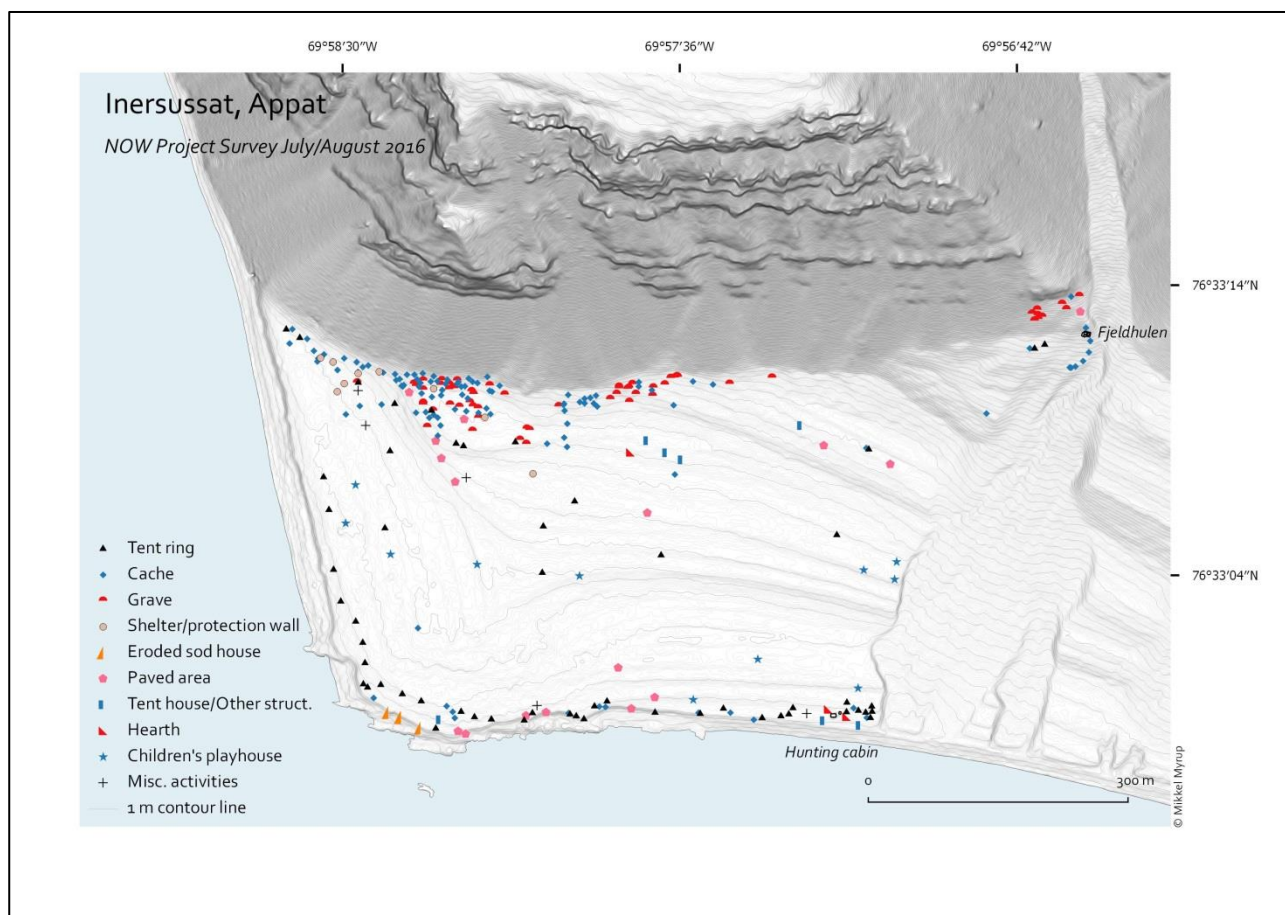
Fig. 4. Topografisk kort over Inersussat-bopladsen på Appat (Nunniffiit nr. 3954), baseret på fotos fra overflyvning med fastvinge-drone. Anlæggene er indplottet ud fra data fra håndholdt GPS. (Kort: Mikkel Myrup, Grønlands Nationalmuseum og Arkiv).
