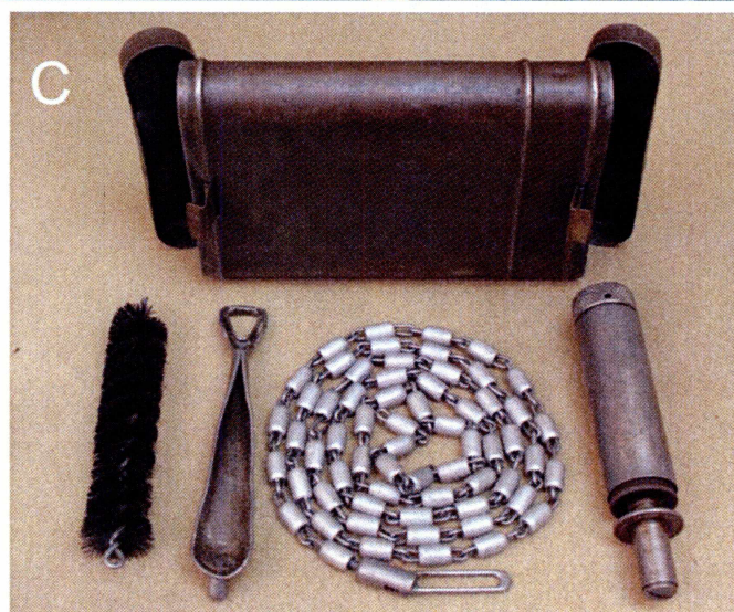
Fig 82. Reinigungsgerät 34, rensesæt. A og B viser rusten blikdåse med rensesæt i Neue Hütte, ved B er den rustne dåse vippet til siden. C viser et komplet sæt. Kæden til at trække gennem piben er af aluminium, hvorfor den i modsætning til dåsen på A og B ikke er rusten, men irret hvid af aluminium oxyd.
