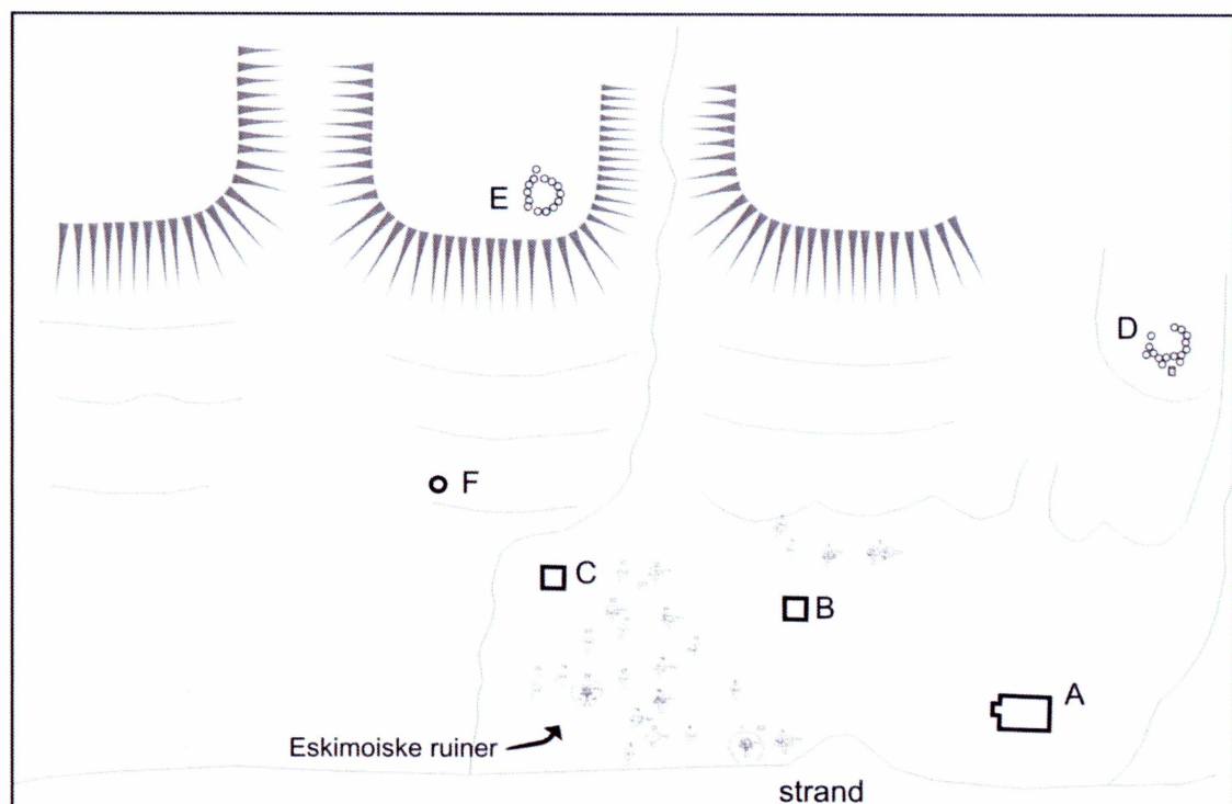
Fig. 55. Skitse over placeringen af Slædepatruljens stationshus, i relation til udhuse, skydestillinger og eskimoiske ruiner.
