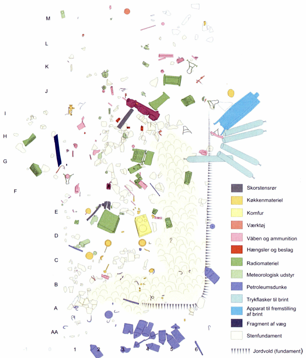
Fig. 73. Udvalgte objekter i brandtomten af Alte Hütte. Efterladenskaberne domineres af trykflasker til brint, og petroleumsdunke stod opmagasineret langs husets ydervægge, men komfuret og radioarmaturer springer også i øjnene. Huset var bygget på et fundament af basaltsten.
