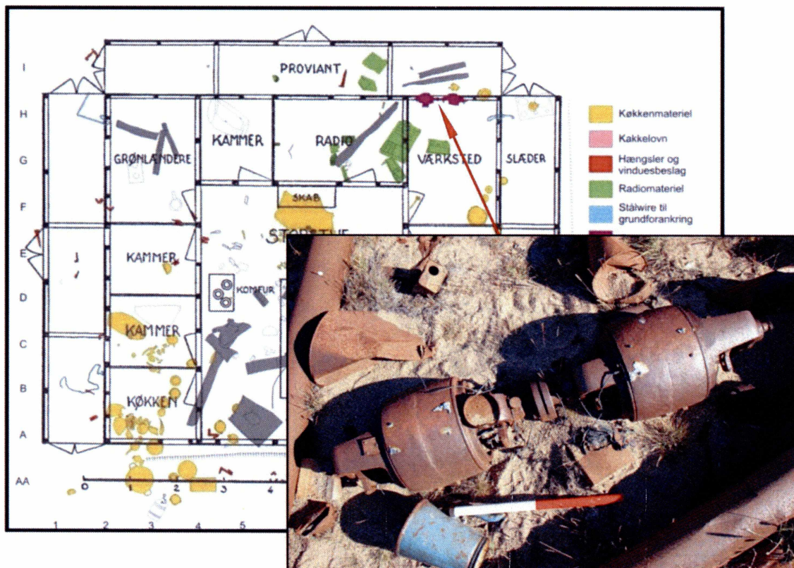
Fig. 12. Generatoren ligger i værkstedet, nær det sted den oprindelig var placeret.
